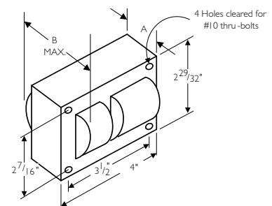
Fig. 14 (3" x 4" Core)
